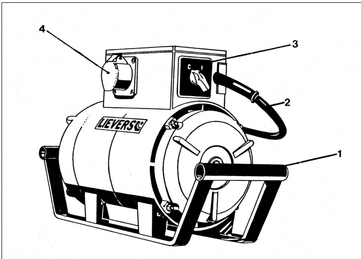
Figuur 1 Overzicht belangrijkste componenten
